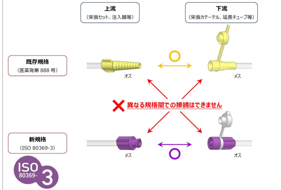
図 1 既存規格と新規格の形状の違い
